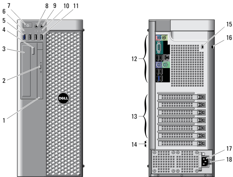
Figur 1. Set forfra og bagfra
